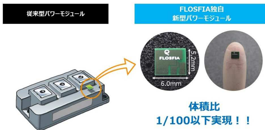
図1：FLOSFIA 独自 新型パワーモジュールと従来型パワーモジュール
